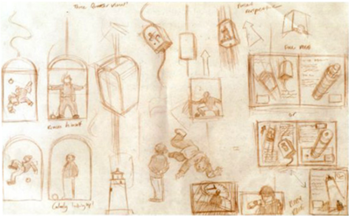
Atracción gravitatoria
