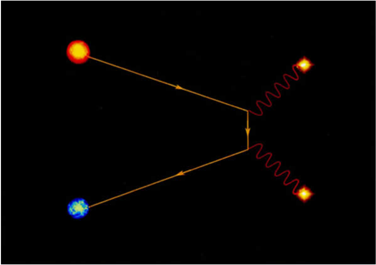
Diagrama de Feynman en teoría de campos
