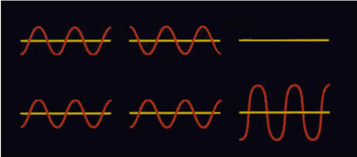
En fase y oposición de fase
