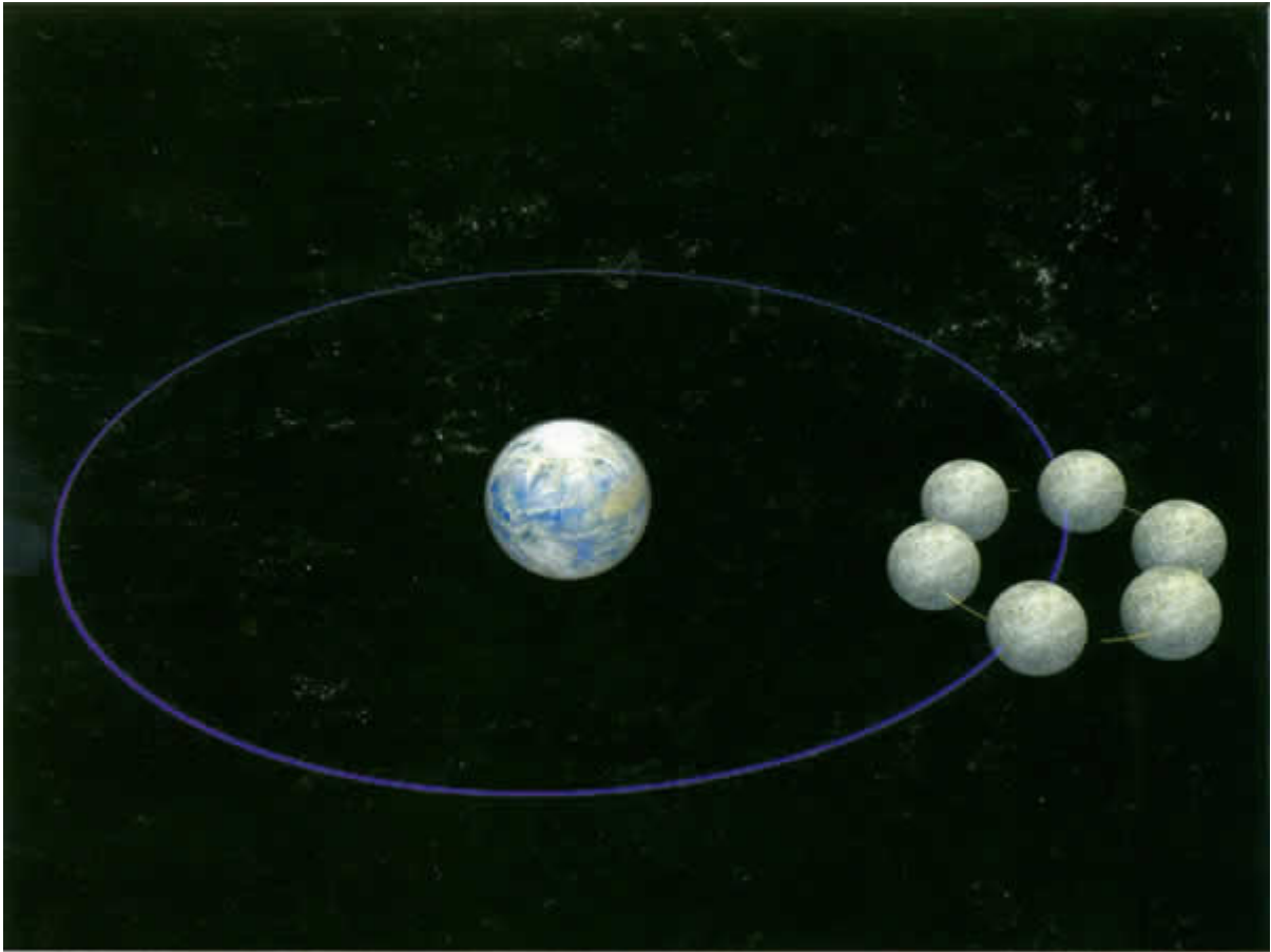
Epíclidos en el modelo de Ptolomeo
