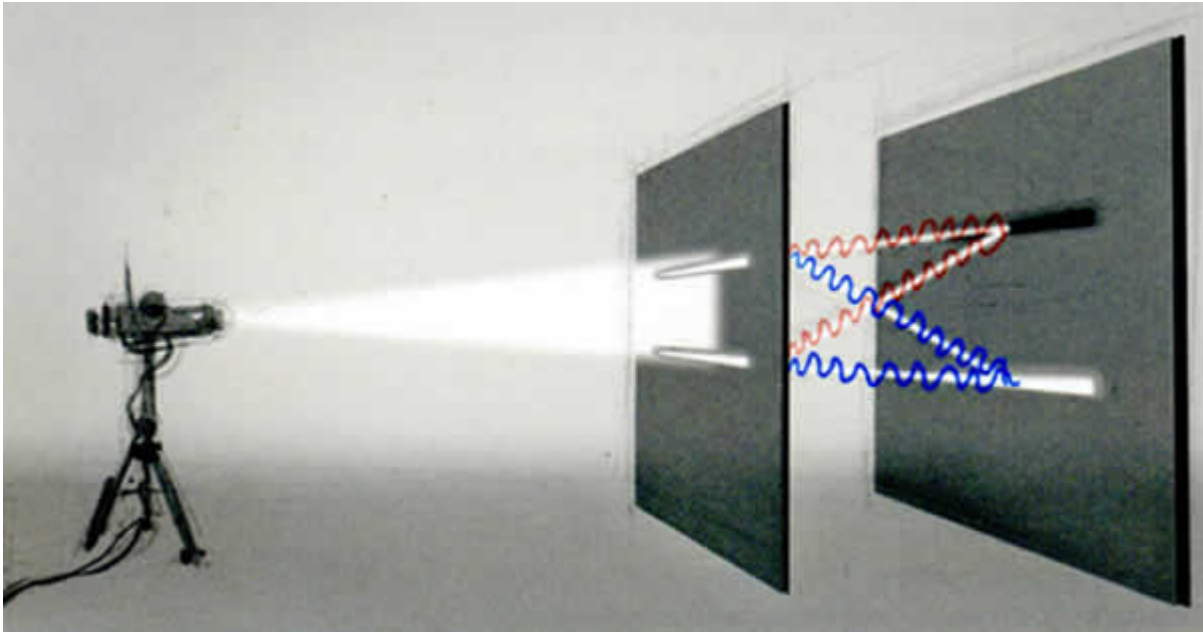
Distancias recorridas e interferencia
