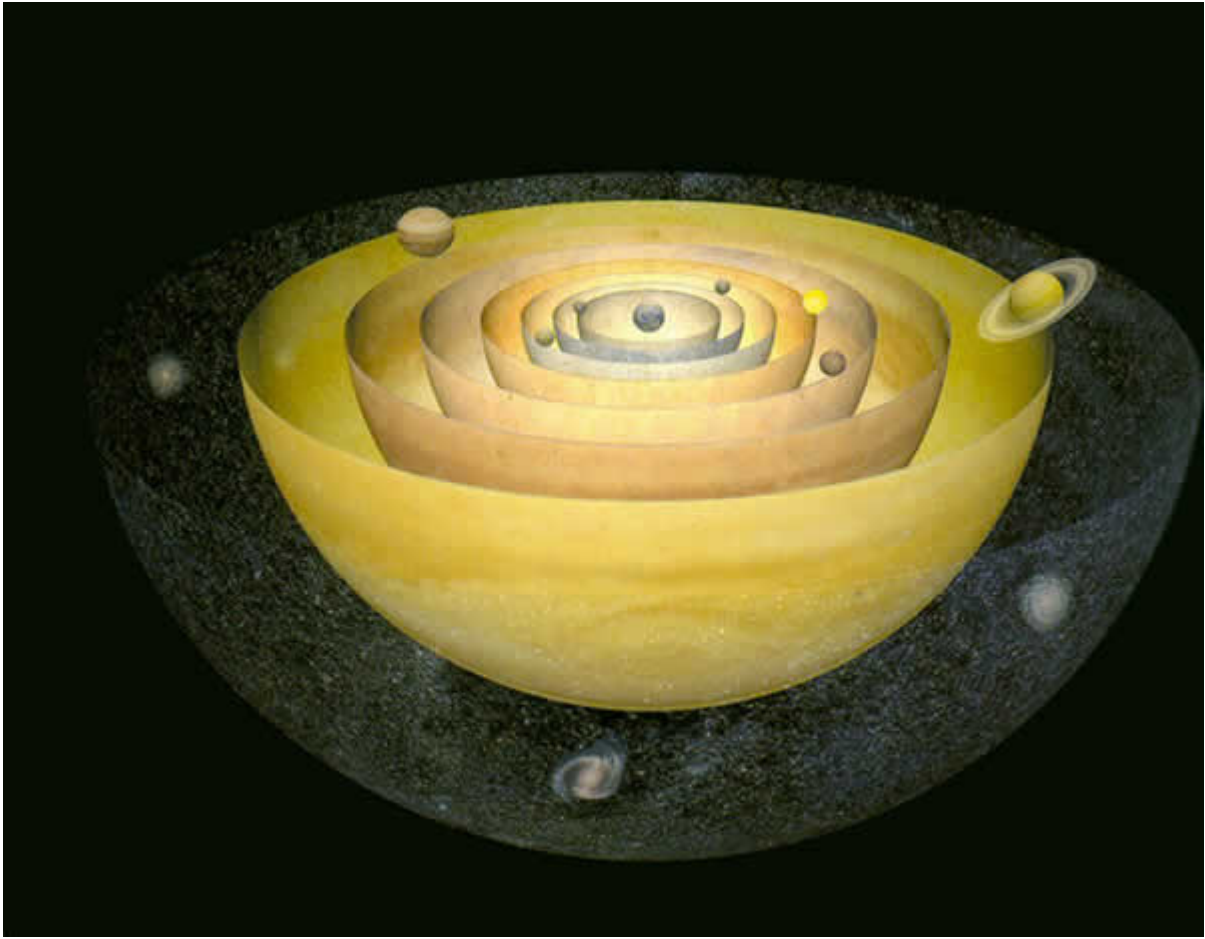
Modelo de Ptolomeo
