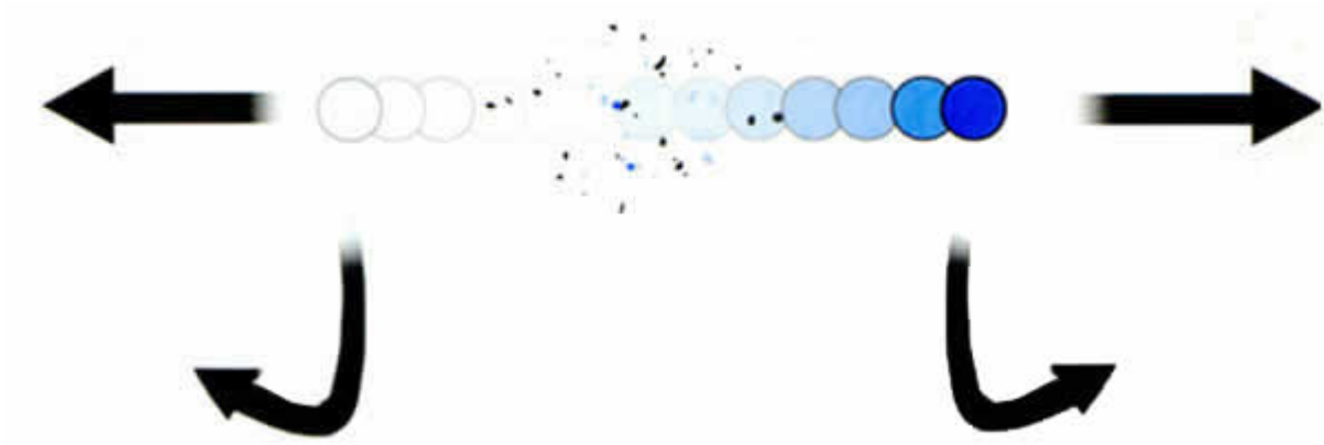
Par electrón/positrón producido por un fotón energético
