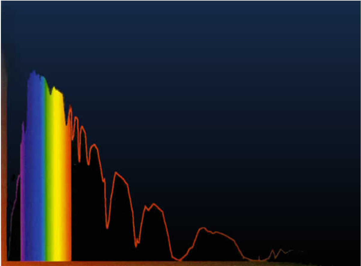
Espectro estelar
