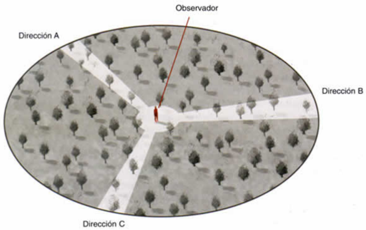
Bosque isotrópico
