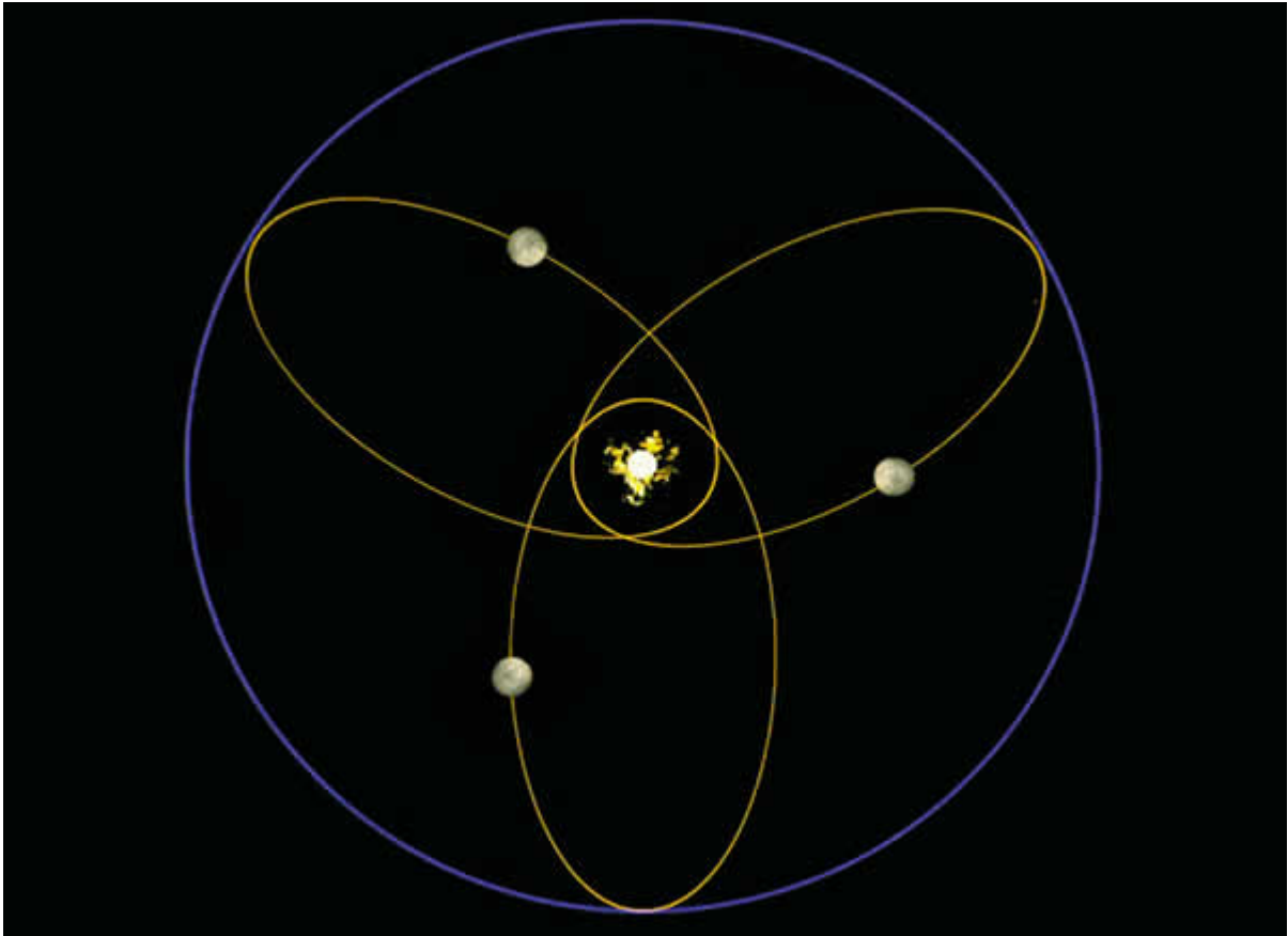
Precesión de la órbita de Mercurio
