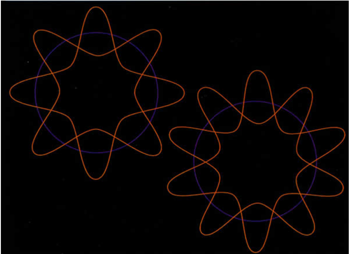
Ondas en las órbitas atómicas
