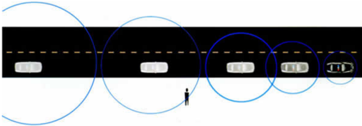
El efecto Doppler
