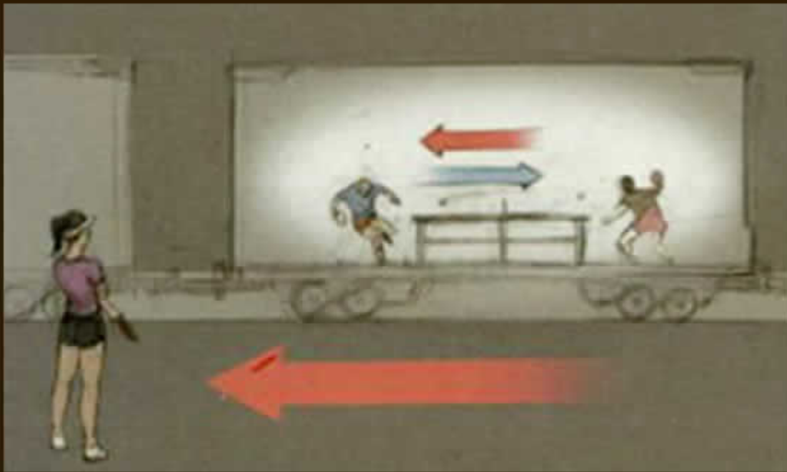
Las diferentes velocidades de la pelota de ping-pong
