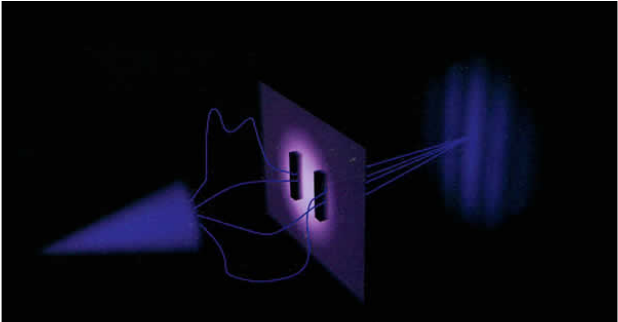
Caminos de electrones que interfieren
