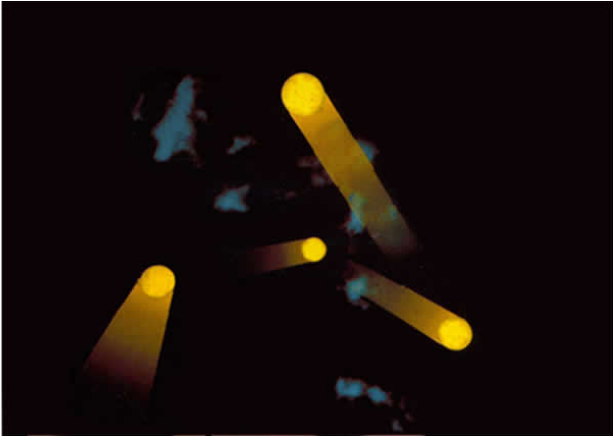
Posición cuántica difuminada
