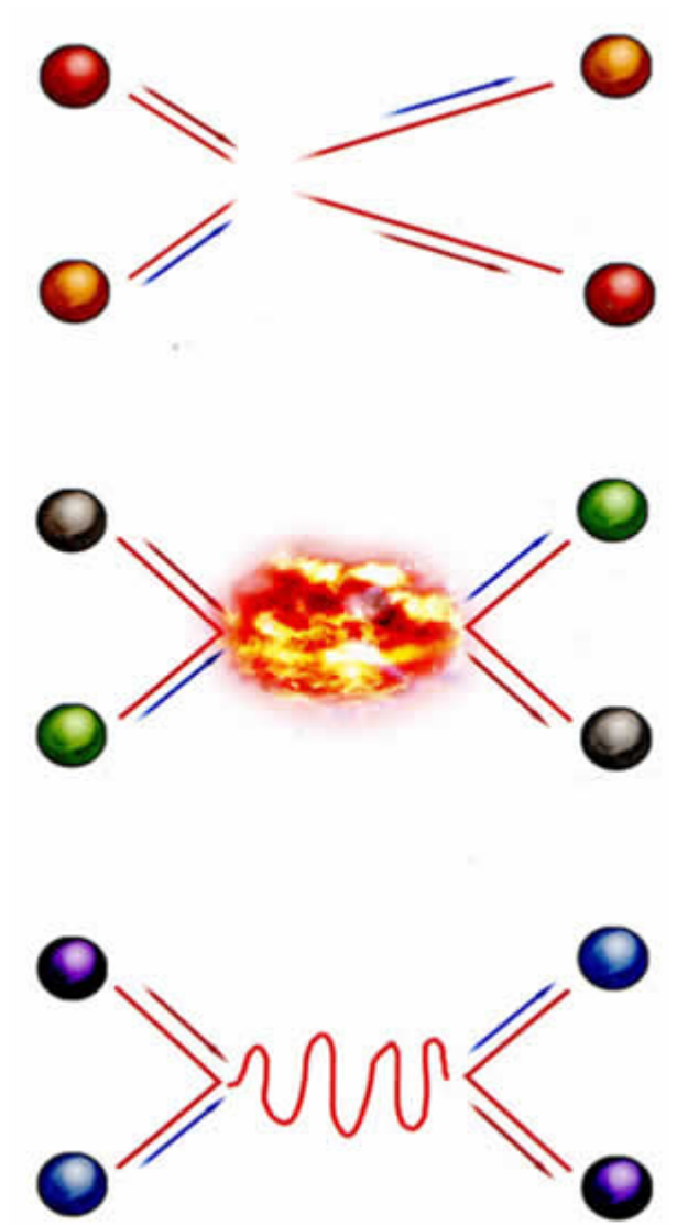
Intercambio de partículas
