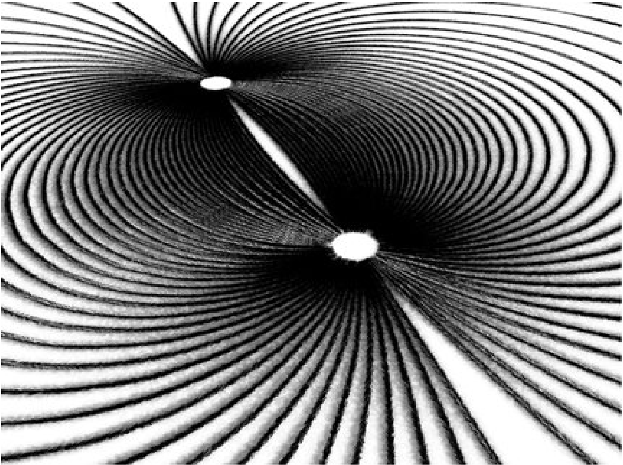
Campos de fuerza. Campo de fuerza de un imán rectilíneo, visualizado mediante su reacción sobre las limaduras de hierro.
