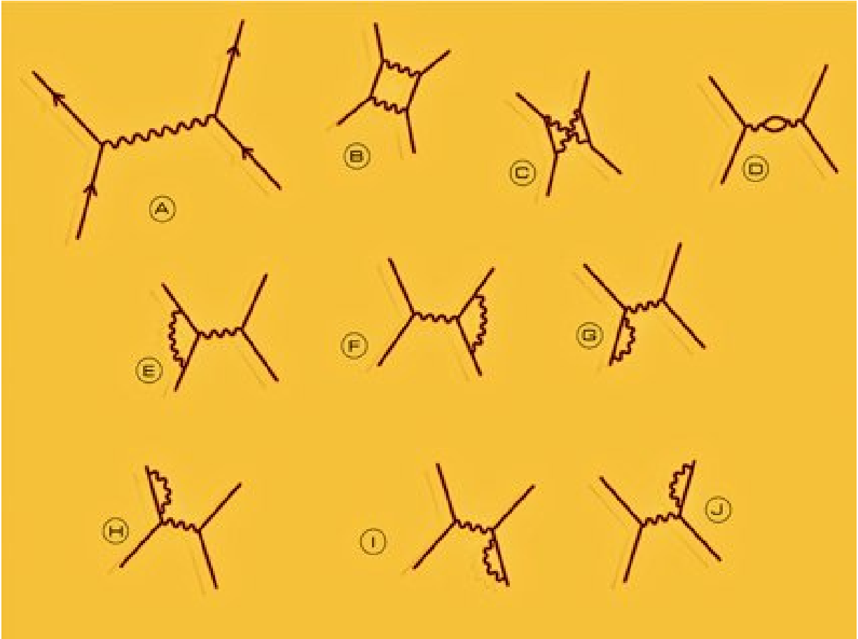
Diagramas de Feynman. Estos diagramas corresponden a un proceso en que dos electrones se desvían uno al otro.
