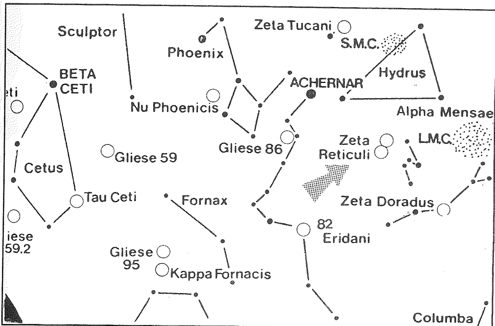
Arriba: mapa estelar que muestra a Zeta Reticuli, visible desde el hemisferio sur.
