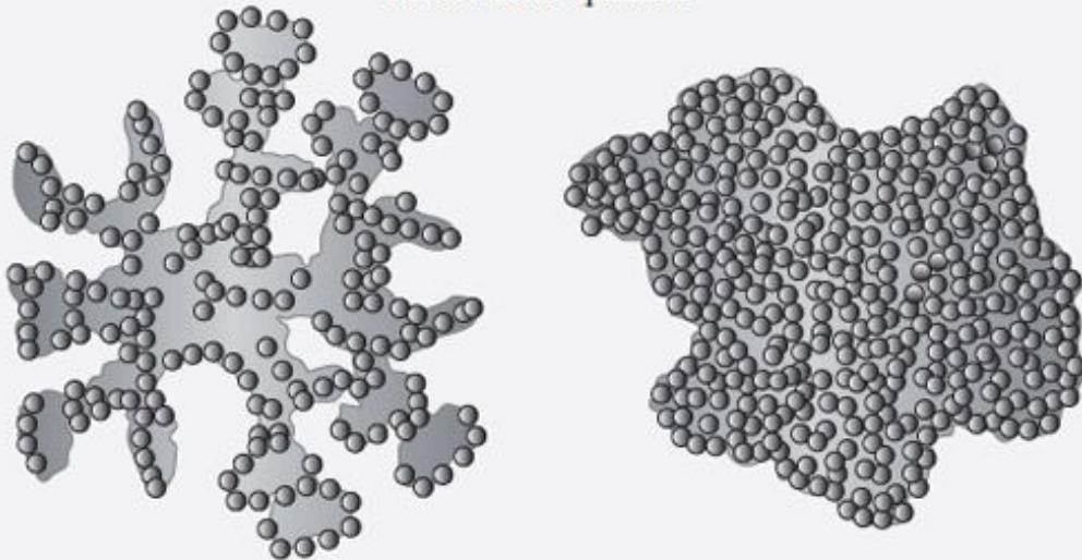
Reticulación química
