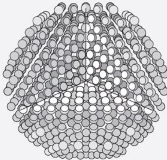
Reticulación electroquímica
