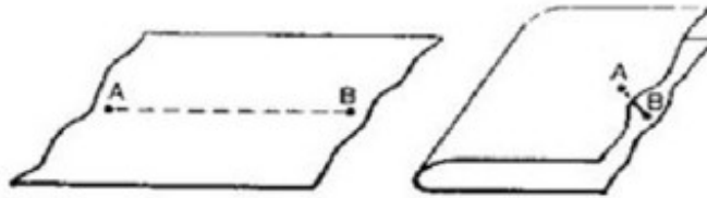
Figura 23. Sentido geométrico del método fantástico de la transportación cero
