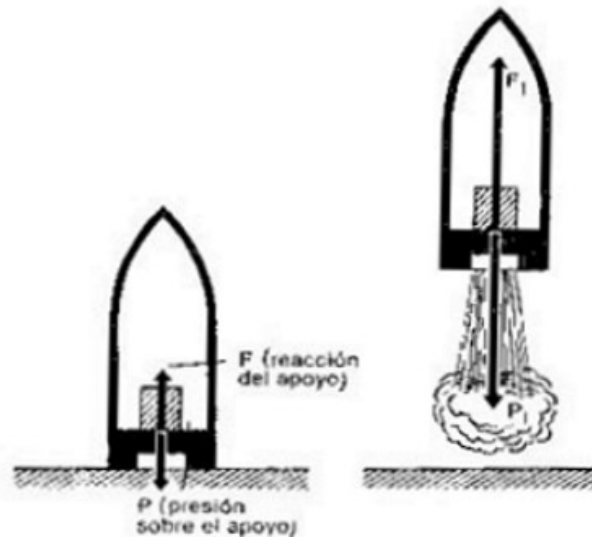
Figura 18. Esencia física de la sobrecarga
