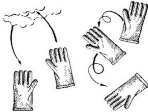
Figura 22. Experimento con el guante
