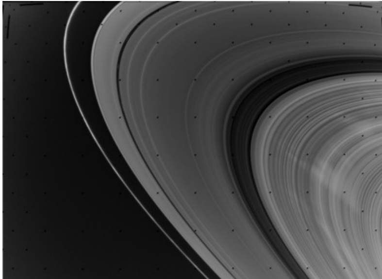
Figura 9. Anillos de Saturno (Foto tomada por la sonda cósmico "Voyager-1".)
