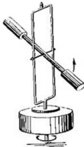
Figura 4. Péndulo de Poshejonov
