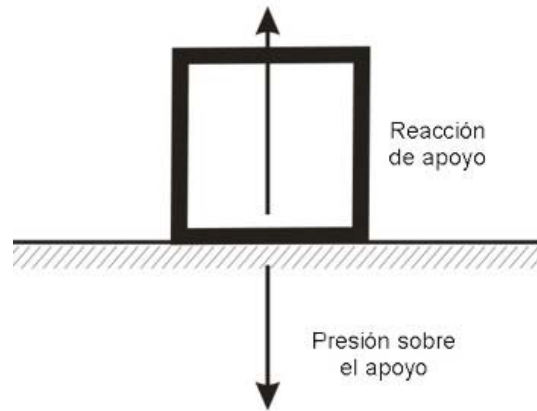
Figura 17. Presión sobre el apoyo y reacción del apoyo
