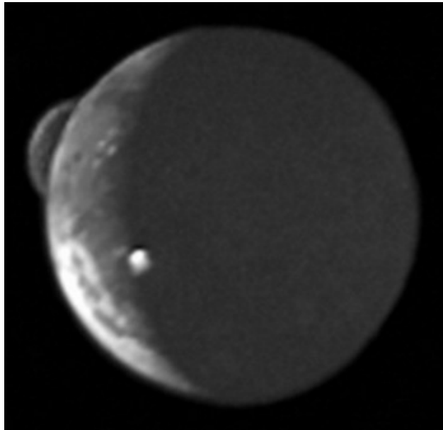
Figura 10. Erupción de un volcán en el satélite de Júpiter, Io. (Foto tomada por la sonda cósmica "Voyager-1").
