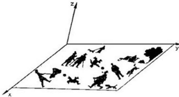
Figura 20. Seres bidimensionales imaginarios
