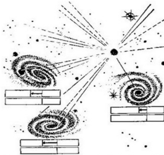
Figura 14. Esquema de la expansión de la Metagalaxia. El desplazamiento hacia el rojo de las líneas espectrales aumenta con la distancia
