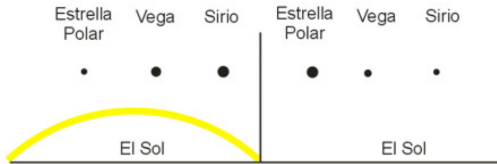
Figura 1. Luminosidad visible de las estrellas, en función de la distancia
