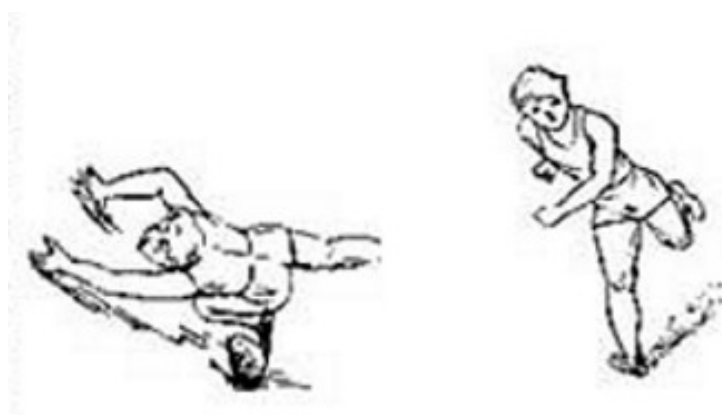
Figura 12. Ilustración aparente de la primera ley de Newton
