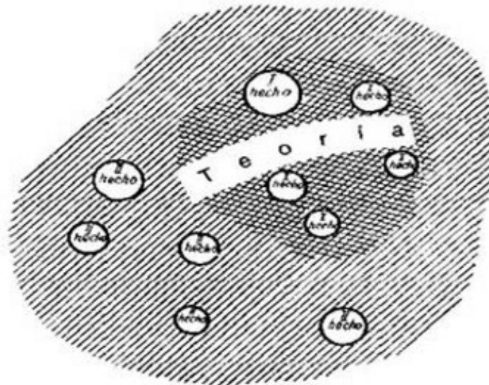
Figura 3 . Desarrollo del conocimiento de la teoría particular a la general
