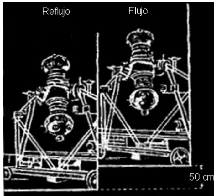
Figura 13. El valor de la marea lunar en le materia sólida de la Tierra en la región de Moscú
