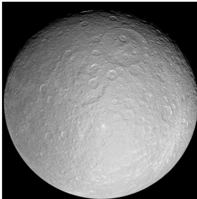
Figura 7. Rea, satélite de Saturno, fotografía tomada por la Voyager-1
