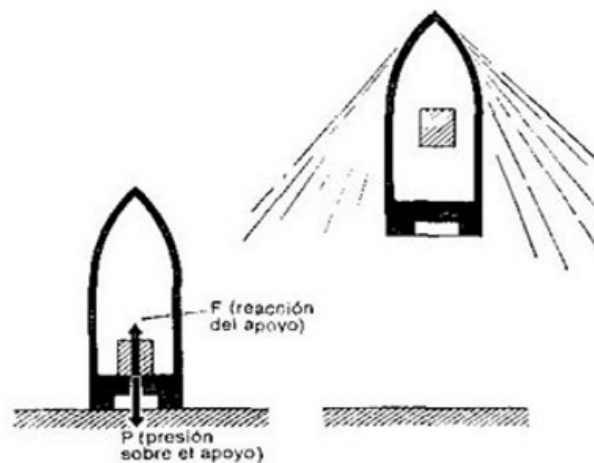
Figura 19. Esencia física de la imponderabilidad
