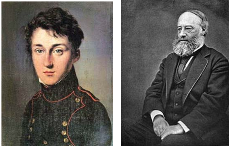
Nicolas Leonard Sadi Carnot (1796-1832) y James Prescott Joule (1818 - 1889)
