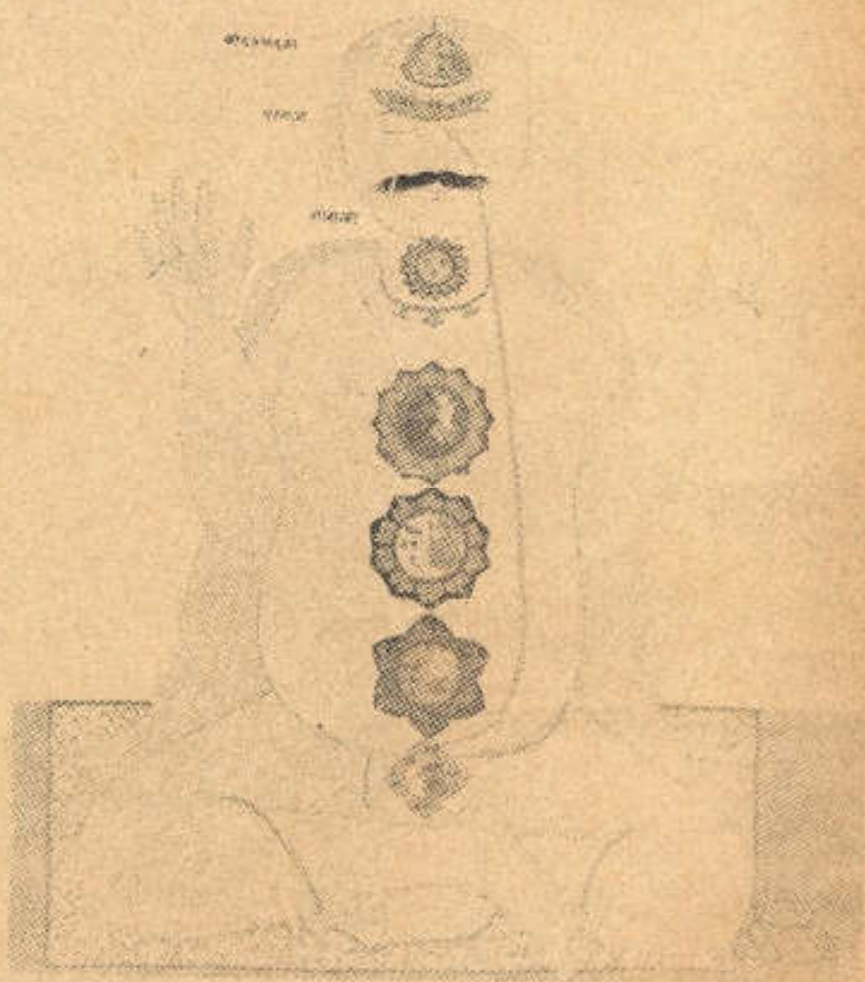
Diagrama del sistema de canales y chakras en el cuerpo sutil (siglo XIX).
